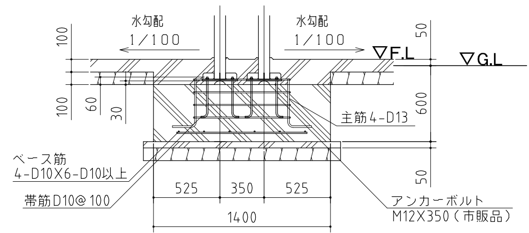
A-A' 断面
